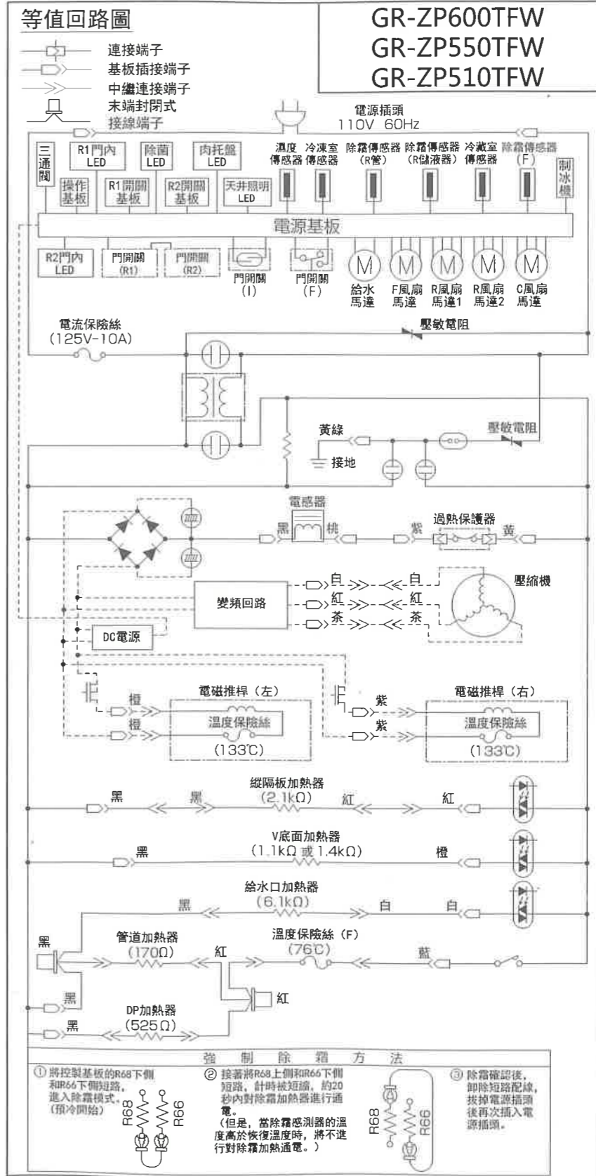
東芝冰箱配線圖
