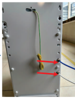
8. Lắp ống nhựa PE từ van cấp nước đến ngõ vào nước trên máy, rồi lắp thêm ống cho ngõ xả nước.
