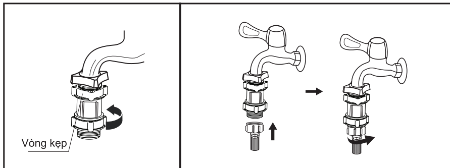
Lắp đầu bộ lọc vào vòi nước và siết chặt vòng kẹp
