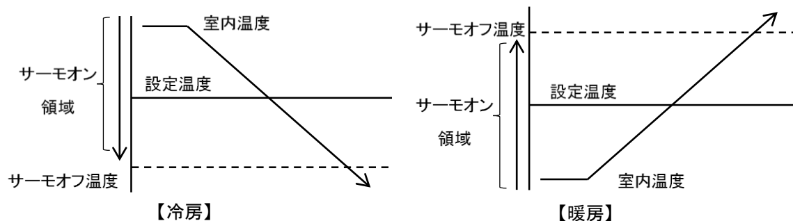
図 3： 動作確認試験における室内温度変化 (冷房および暖房)
