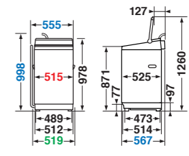
◎寸法図【AW-7DH2/6DH2 共通】
