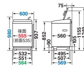
◎寸法図【AW-9DH2/8DH2 共通】
