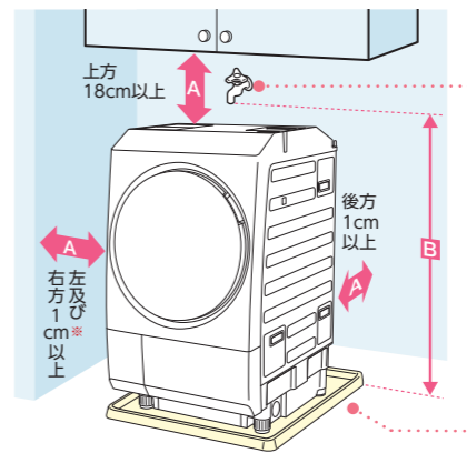
*排水ホースが通る側は10cm以上。
