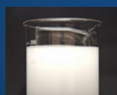
マイクロバブルが入った 水は白く濁る。
