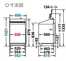
◎寸法図
