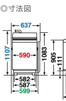
◎寸法図
