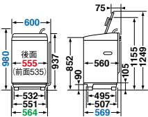
◎寸法図【AW-9DH5/8DH5 共通】
