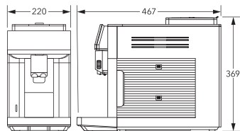
寸法図
